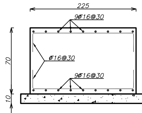
Section D-D
